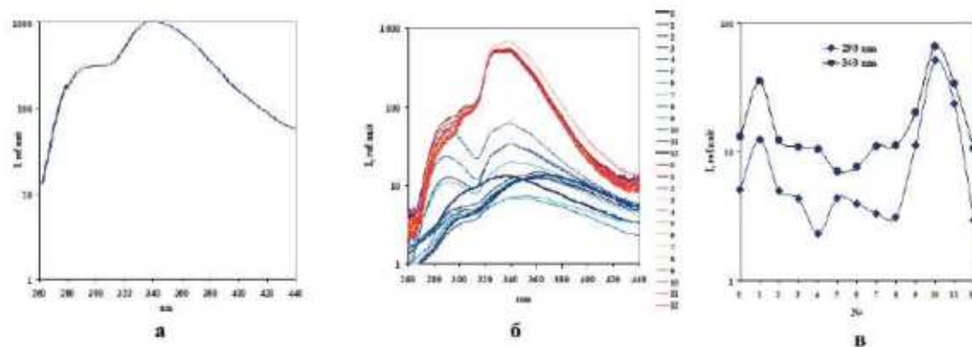
Рис.1. Спектр люминесценции в интервале длин волн 260 – 440 нм (возбуждение \lambda=220 нм) раствора АТ ИФНг ( C_0 = 2.5 мг/мл) в глициновом буфере (а). Спектры люминесценции в интервале длин волн 260 – 440 нм (возбуждение \lambda=228 нм) В/ВС растворов АТ ИФНг для разбавлений C_1-C_{12} (серия 1), нижняя группа спектров (оттенки синего цвета) относится к водным растворам, верхняя (оттенки красного цвета) – к водно-спиртовым растворам (б). Максимумы интенсивности люминесценции на длинах волн 290 и 340 нм для водных растворов АТ ИФНг (серия 1) от номера разбавления (в). Все графики представлены в полулогарифмических координатах
