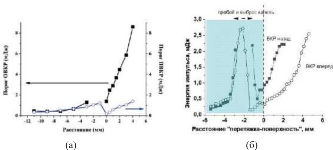
Рис. 1. N-образная зависимость порога ВКР в лёгкой H_2O (а) и тяжёлой D_2O (б) воде: попутный ВКР (вперёд, круги) и обратный ВКР (назад, квадраты).
