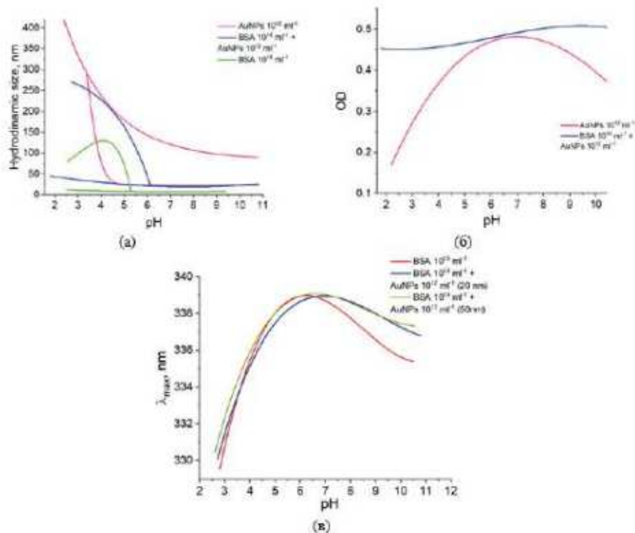
Рис.1. Влияние кислотности среды на физические характеристики коллоидных растворов BSA (10 16 ml -1 ), AuNPs 8nm (10 12 mL -1 ), BSA (10 16 ml -1 ) + AuNPs 8nm (10 12 mL -1 ): (а) распределение частиц по размерам, (б) максимум поглощения, (в) длина волны максимума флуоресценции
