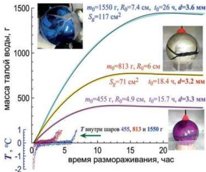
Рис. 1 Кинетики накопления талой воды в ходе таяния шаров разной начальной массы. Сплошные кривые показывают фитирование экспериментальных данных с использованием предложенной модели. При обработке данных также учитывалось, что в первые 10-20 мин лёд прогревался от температуры морозильной камеры до температуры плавления. При этом образование талой воды еще не началось. Внизу показаны зависимости температуры внутри ледяных шаров, измеренные термодатчиком DS18B20. Видно, что в процессе плавления температура внутри шаров равнялась 0 °С. Последующий рост температуры связан с выходом термодатчика из объема шара на его поверхность и наличием контакта с теплым воздухом.
