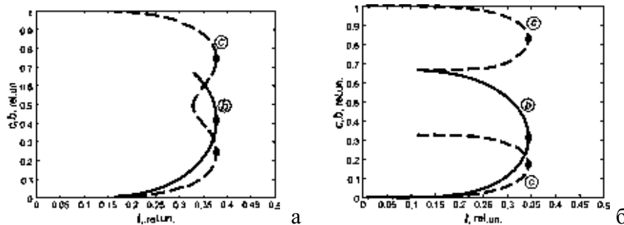
Рис. 1. Температурные зависимости концентраций c (штриховые линии) и b (сплошные) при энергиях водородных связей, D , равных 0.7 (а) и 1.0 (б). Черные кружки - критические точки.
