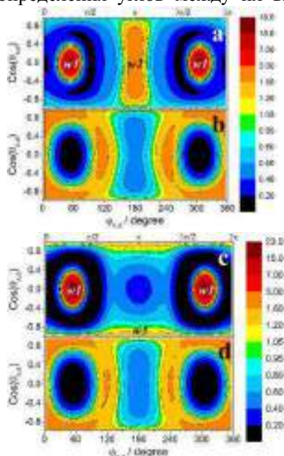
Рис.1 Распределения ориентаций молекул воды в сферических угловых координатах, описывающих направление на органику относительно вектора нормали \mathbf{n} и дипольного момента \mathbf{d} вблизи белка (a,b) и мембраны (c,d) в первой (a,c) и второй (b,d) оболочках.
