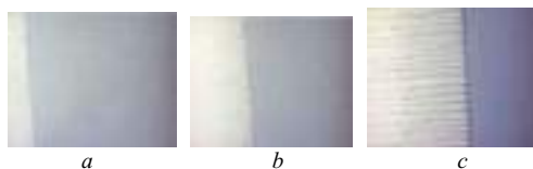
Рис. 1 Формирование периодической структуры при кристаллизации раствора.
