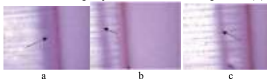
Рис. 3. Экстремум концентрации компонента между жидкой и твердой фазами раствора (показан стрелками).
