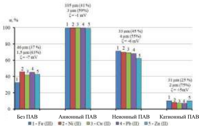
Рисунок 1. Влияние ПАВ анионного, катионного и неионного типов на поверхностные характеристики и степень извлечения суммы малорастворимых соединений металлов, pH = 9,5 – 10,5; \tau процесса = 10 мин.; i_c = 0,4 А/л.
