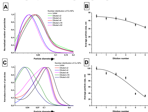
Рис.1 Нормированные распределения числа частиц по размеру и зависимость среднего размера частиц от числа разбавлений в случае: (A), (B) наночастиц железа; (C), (D) – наночастиц меди.
