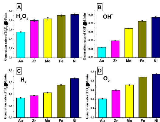
РИС.1. Влияние материала наночастиц на процессы генерации. (А) - скорость генерации перекиси водорода, (В) - скорость генерации гидроксильных радикалов, (С) - скорость генерации молекулярного водорода, (D) - скорость генерации молекулярного кислорода.
