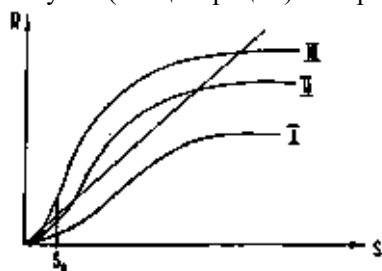
Рис.1. Кривая I лежит ниже порога распространения возбуждения, кривая II, начиная с определенного уровня стимула, превосходит порог, а кривая III имеет порог ниже определяемого уровнем шумовых стимулов ( S_0 ).
