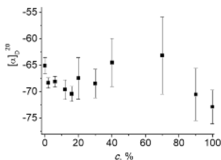
Рис. 1. Удельное вращение 0.1 М растворов левоглюкозана в смесях ДМСО–вода с содержанием ДМСО 0–100 мол.% (среднее значение для каждой концентрации ДМСО, 3 раствора). Ошибку рассчитывали, как стандартное отклонение от среднего ( p = 0.05 ).
