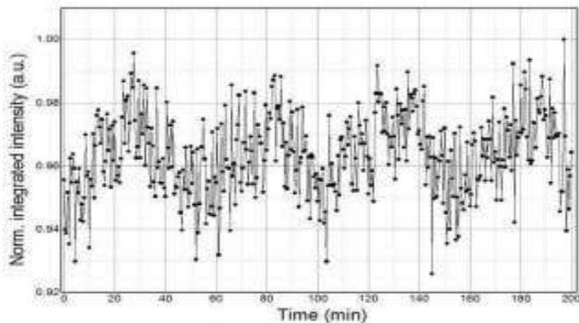
Рис. 1. Динамика интегральной интенсивности ЯМР сигнала в магнитном поле Земли [1].
