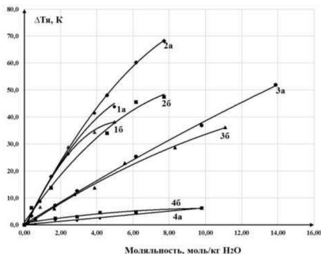
Рис. Разность радиоярких температур растворов – вода по расчетным (а) и экспериментальным (б) данным на частоте 61.2 ГГц. Растворы: 1а, 1б – диметилформамид; 2а, 2б – диметилацетамид; 3а, 3б – ацетамид; 4а, 4б – формаимид.
