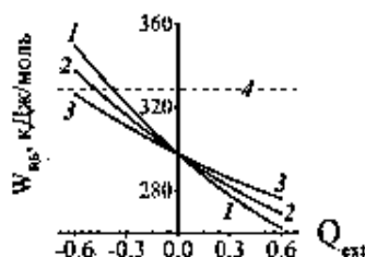
Рис. Зависимость энергии сольватации W для \text{Rb}^+ рассчитана по (2)-(5) (при корреляционной длине \lambda_3 = 3\text{\AA} ) как функция части заряда катиона Q_{\text{ext}} , локализованного за пределами борновской сферы катиона. Значения параметра \eta в (4) для линий 1,2,3: \eta = 0.5, 0.4, 0.3 . Радиус r_i для \text{Rb}^+ взят по шкале Гуарри и Адриана: 1.63\text{\AA} . Линия 4 соответствует экспериментальным данным для \text{Rb}^+ [5].
